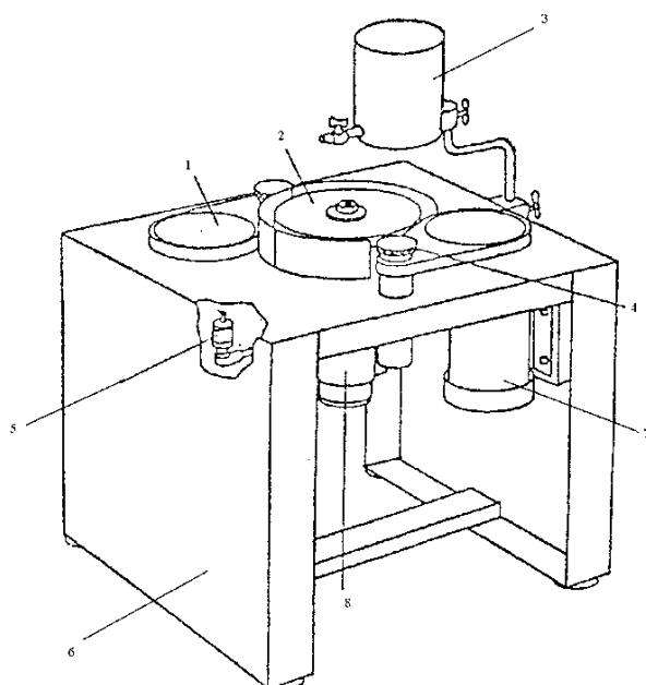
Рис. 2 Модель FAC-10А. Шпиндель с четырёхступенчатым переключением скоростей. 1-Стол гранитного устройства; 2- Планшайба; 3- Капельник для подачи СОЖ; 4-Микрометрическая шкала; 5- Маслёнка; 6- Рама корпуса; 7- Эл. Двигатель; 8- Шпиндель.
