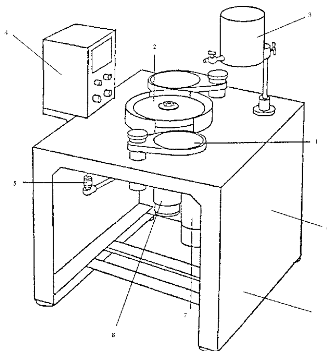
Рис. 3 Модель FAC-10В. Шпиндель с бесступенчатым переключением скоростей. 1-Стол гранитного устройства; 2- Планшайба; 3- Капельник для подачи СОЖ; 4-Регулятор скорости; 5- Маслёнка; 6- Рама корпуса; 7- Эл. Двигатель; 8- Шпиндель.
