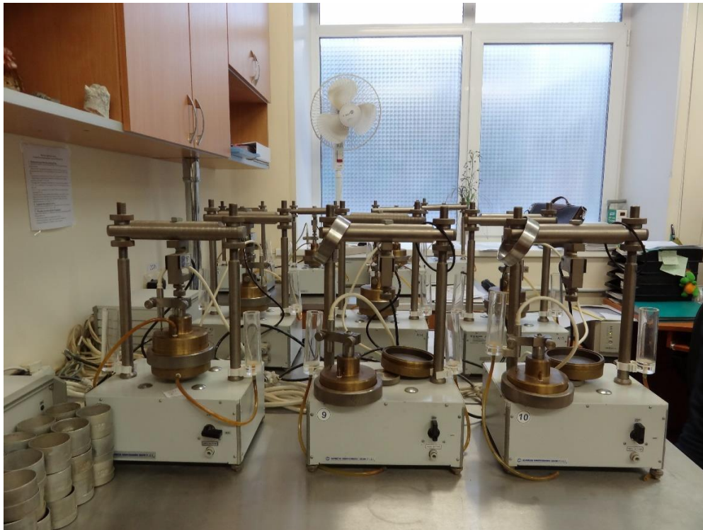
Рис. 1.5 Компрессионные приборы [8, с. 46]
