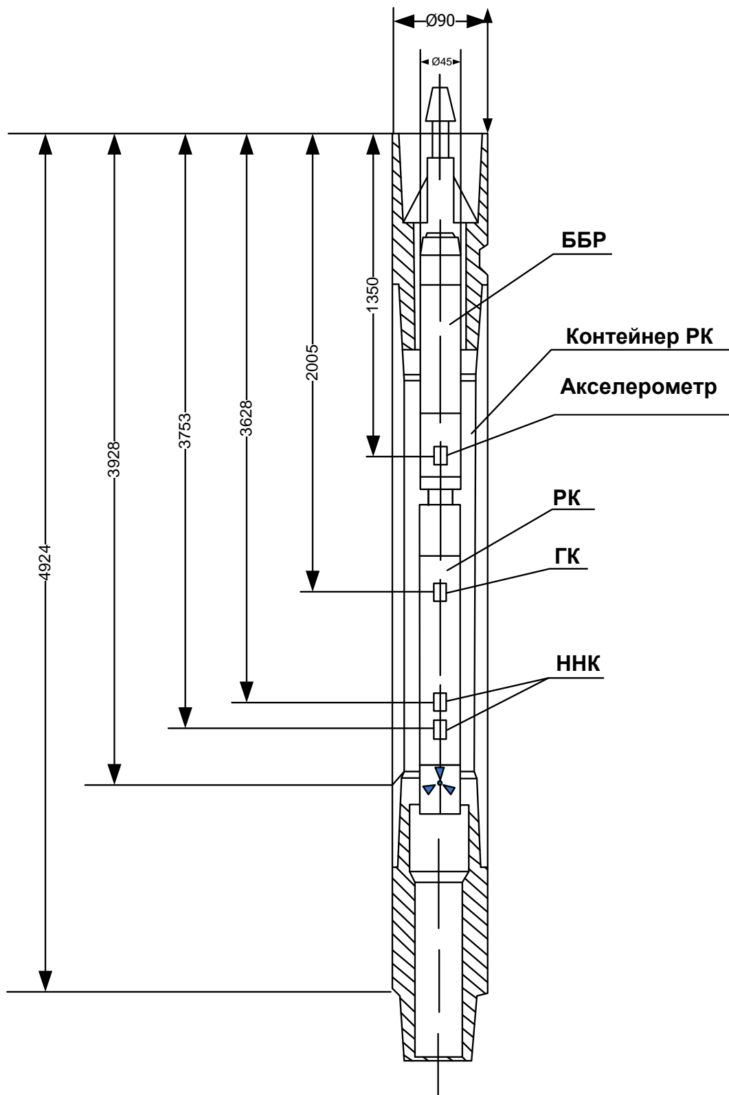
Рис. 5.2. Прибор РК
