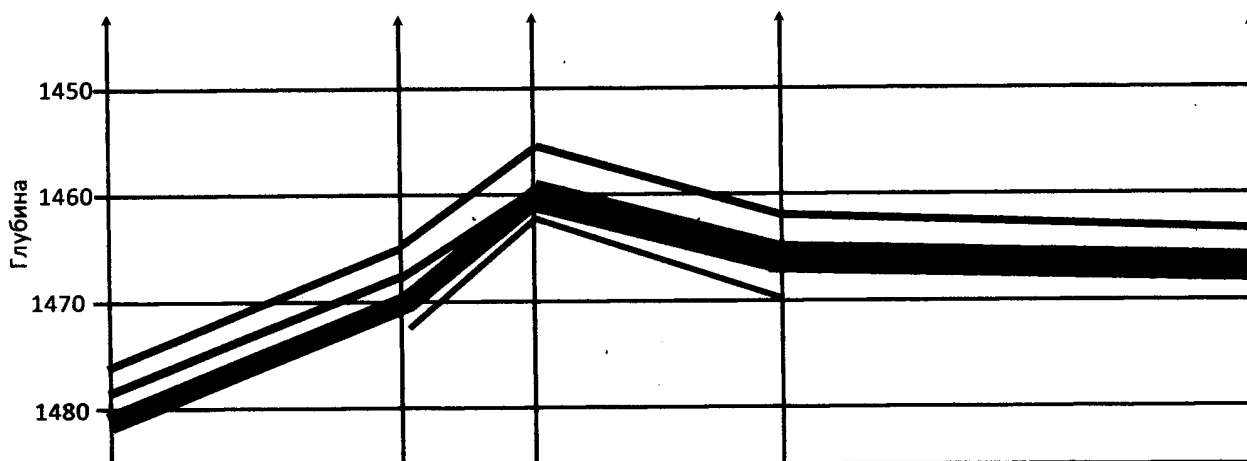
Рис. 7.3. Корреляционный разрез
