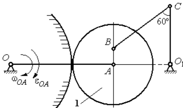
Рис. 2.36. Механизм качалки
