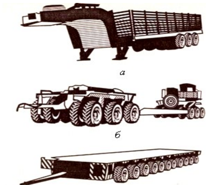
Рис. 19. Полуприцеп и прицепы-тяжеловозы грузоподъемностью: a — 52 т; б — 120 т; в — 300 т
