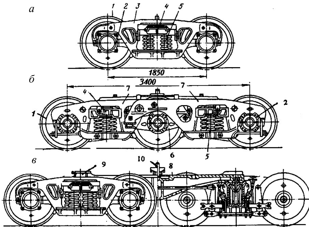
Рис. 3. Вагонные двух- (а), трех- (б) и четырехосные (в) тележки: 1 – колесная пара; 2 – букса; 3 – боковая рама; 4 – надрессорная балка; 5 – рессорные комплекты; 6 – балансиры; 7 – боковая полурама; 8 – соединительная балка; 9 – подпятник соединительной балки; 10 – подпятник для кузова
