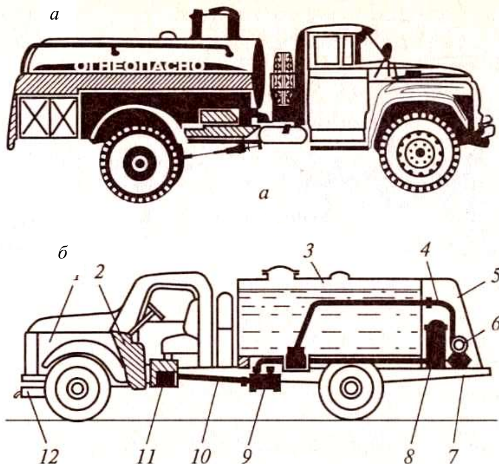
Рис. 12. Автоцистерна-заправщик:
