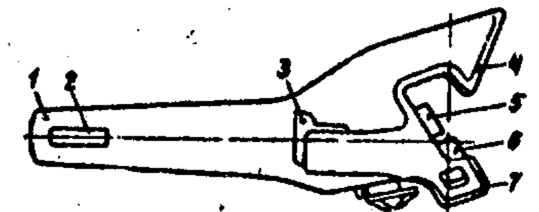
Рис. 2. Корпус автосцепки с механизмом сцепления
