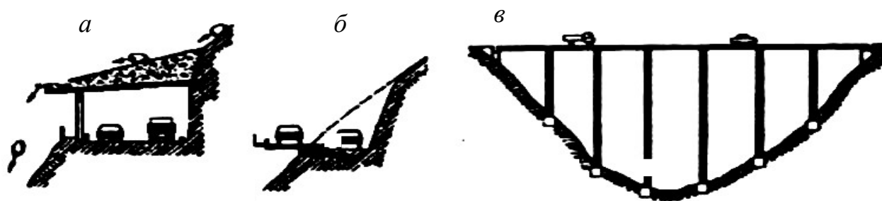
Рис. 6. Искусственные сооружения на горных дорогах: а — галерея; б — балкон; в — виадук
