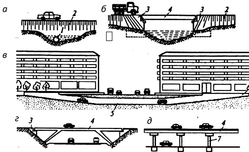
Рис. 5. Основные виды искусственных сооружений: 1 – труба; 2 – насыпь дороги; 3 – устой моста; 4 – пролетное строение; 5 – тоннель; б – парапет; 7 – промежуточная опора
