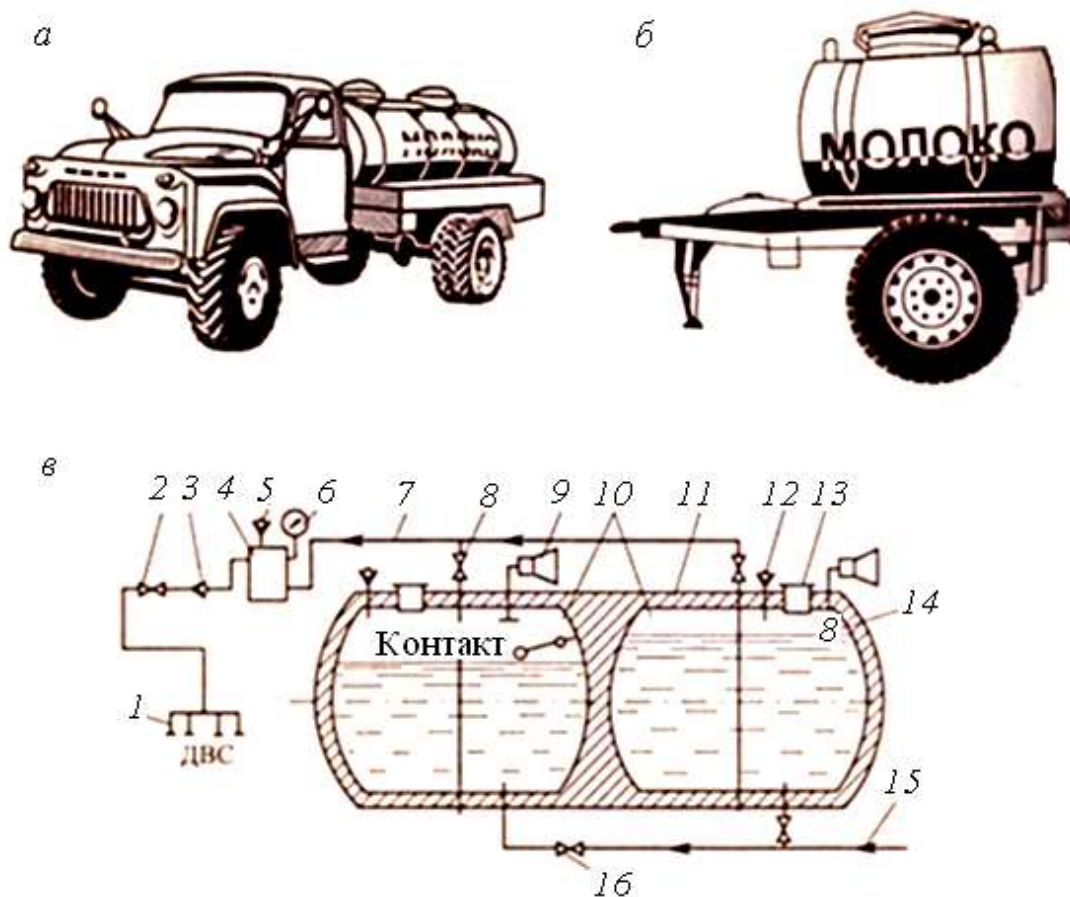
Рис. 13. Цистерны для перевозки молока:
