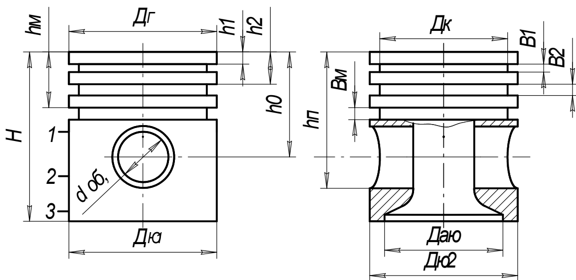
Рис.4. Чертеж поршня
