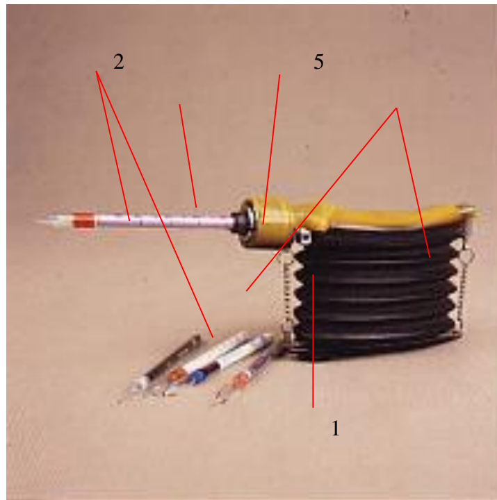
Рис. 16. Газоанализатор GX-4
