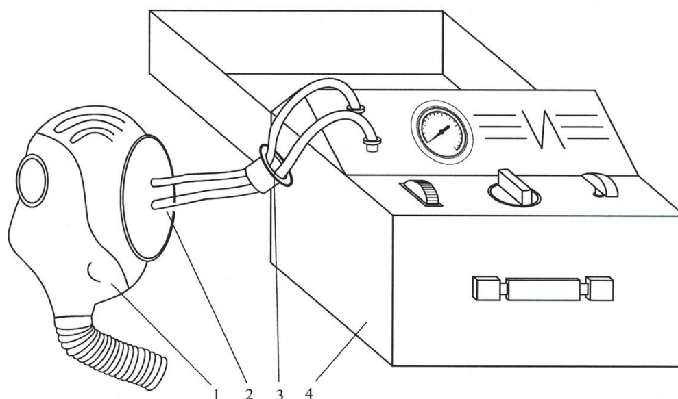
Рис. 5. Схема присоединения респиратора со шлем-маской к индикатору ИР: 1 – шлем-маска; 2 – приспособление для проверки шлем-маски; 3 – фланец овалный присоединительный; 4 – индикатор ИР
