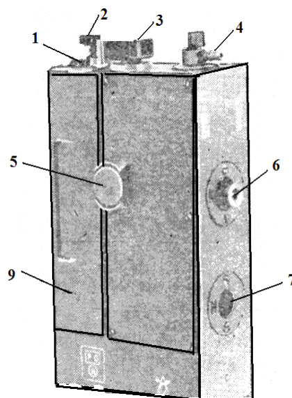
Рис. 6. Общий вид интерферометра
