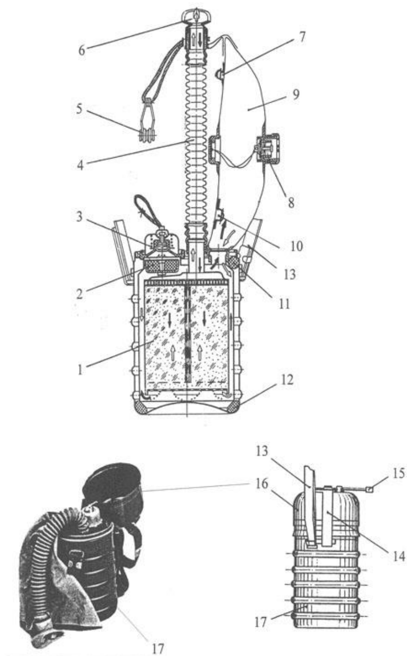
Рис. 7. Самоспасатель ШСС-1М: 1 – патрон; 2 – брикет пусковой; 3 – устройство пусковое; 4 – шланг; 5 – зажим носовой; 6 – загубник; 7 – кнопка; 8 – клапан избыточный; 9 – мешок; 10 – пробка; 11, 12 – амортизатор; 13 – ремень плечевой; 14 – лента; 15 – ремень замка; 16 – крышка; 17 – корпус
