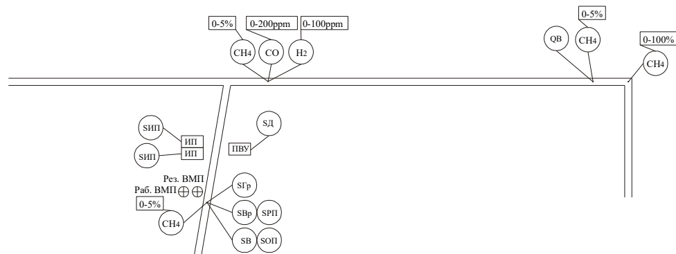
Рис.1.5. Схема расположения аппаратуры СИСТЕМЫ в горных выработках Аналоговые датчики: CH 4 - метана, CO - оксида углерода, O 2 - кислорода, H 2 - водорода, QB - скорости воздуха. Дискретные датчики состояния оборудования: SOK - очистного комбайна, SK - конвейера, SB - вентилятора, SBр - резервного вентилятора, SГр - группового пускателя, SBШ - вентиляционных дверей, СИП - питателя, SY - уровня в бункере, СИП - наличия сетевого питания СИСТЕМЫ, СД - состояния целостности внешней оболочки ПБУ, SPИ - наличия питания резервного вентилятора, SOП - наличия питания основного вентилятора
