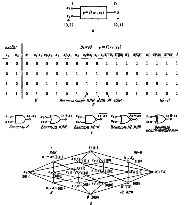
Рис. 2.7. Комбинаторные схемы с двумя входами и одним выходом. а – комбинаторная схема с двумя входами и одним выходом; б – 16 отношений входов и выходов; в – обозначения двухвходовых схем; г – представление последовательности с помощью диаграммы Хассе.
