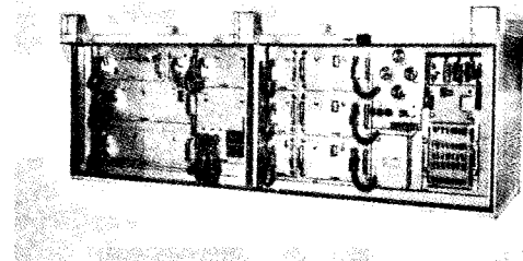
Рис. 3.51. Устройство автовождения с нечетким управлением.
