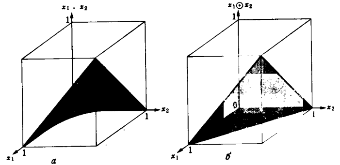
Рис. 2.15. Логическое произведение (x_1 \wedge x_2) .
