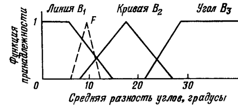
Рис. 3.68. Эталонный образ.
