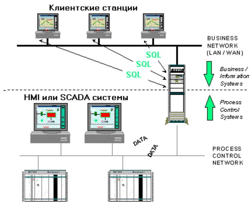
Рис. 3.11. Клиент-серверная организация
