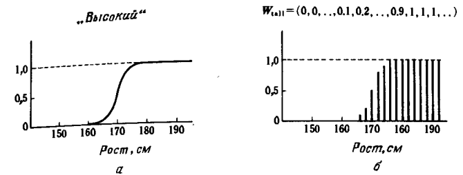
Рис. 6.1. Функция принадлежности, соответствующая слову «высокий», (а) и ее дискретное представление (б).
