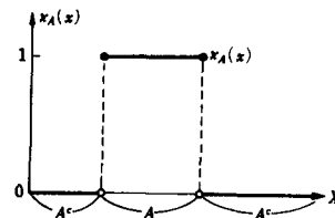
Рис. 2.2. Определение множества с помощью характеристической функции.
