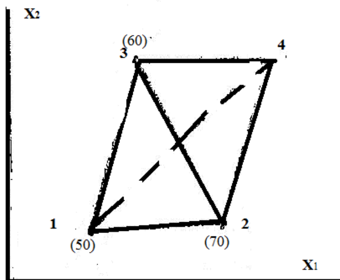
Рис.8.4. Правило отражения
