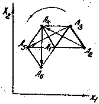
Рис.8.6. Явление заикливания
