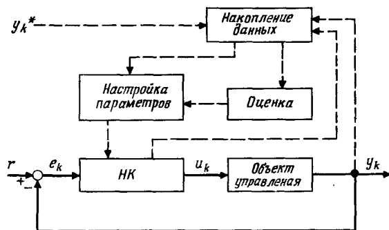
Рис. 3.30. Самонастраивающийся НК.
