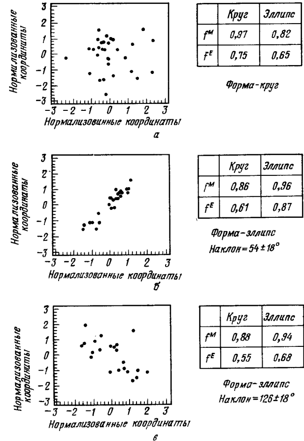
Рис. 3.66. Примеры кластеризации данных. а — PO 2 -HCO 3 ; б — BE-TCO 2 ; в — CU-HB.
