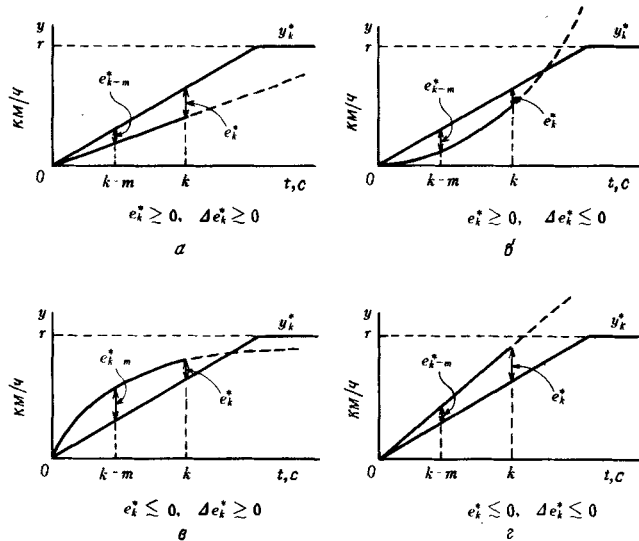
Рис. 3.32. Примеры реакции.
