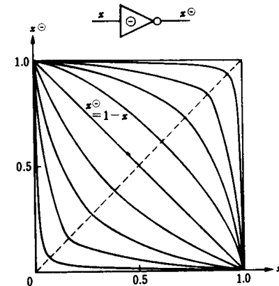
Рис. 2.14. Нечеткие отрицания.
