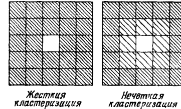
Рис. 3.59. Нечеткая кластеризация.
