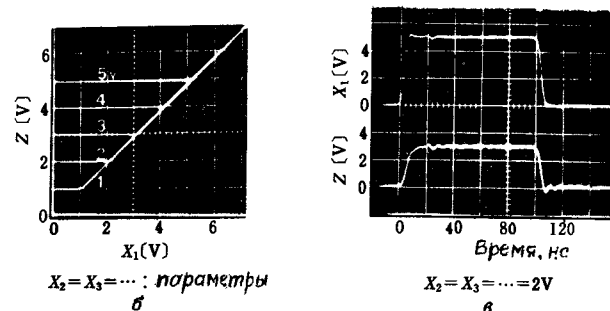
Рис. 6.2. Схема МАХ (а), характеристики входа и выхода (б) и переходная характеристика (в).
