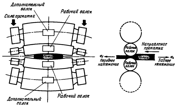
Рис. 3.14. Схема прокатки.
