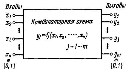
Рис. 2.5. Комбинаторная схема.
