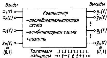
Рис. 2.4. Последовательностная схема.
