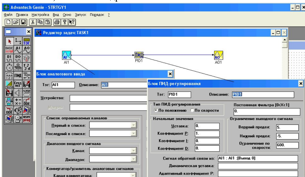
Рис. 34. Задача ПИД-регулятора
