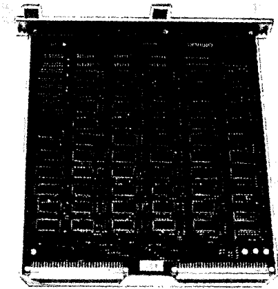
Рис. 6.10. Плата нечетких выводов нечеткого компьютера FUZ-MM1.
