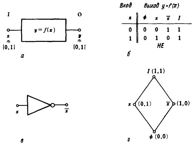
Рис. 2.6. Комбинаторные схемы с одним входом и одним выходом. а – схема с одним входом и одним выходом; б – четыре отношения входа и выхода; в – вентиль НЕ (инвертор); г – представление последовательности с помощью диаграммы Хассе.
