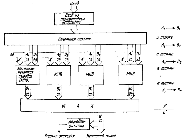
Рис. 6.9. Базовая архитектура нечеткого компьютера.
