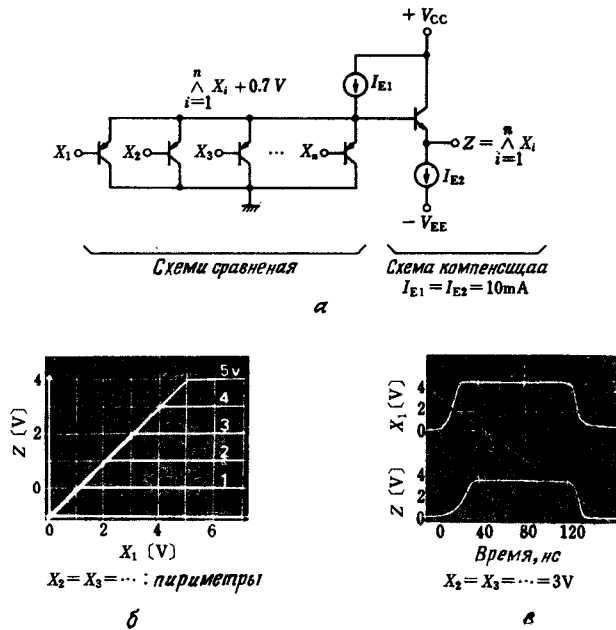
Рис. 6.3. Схема MIN (а), характеристики входа и выхода (б) и переходная характеристика (в).
