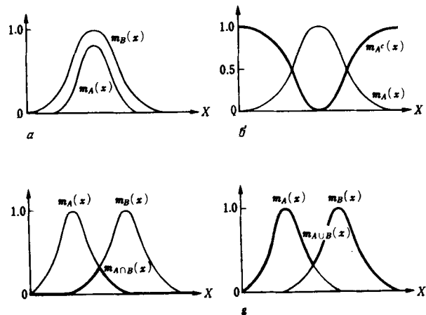
Рис. 2.9. Основные операции над нечеткими множествами.
