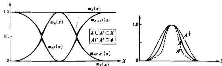
Рис. 2.10. Невыполнение закона Рис. 2.11. Степень \alpha нечеткого множества ( \alpha = 2, 1/2 ).
