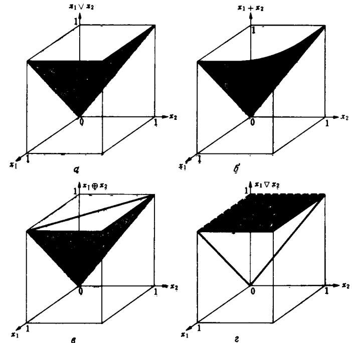
Рис. 2.18. Типичные s -нормы.
