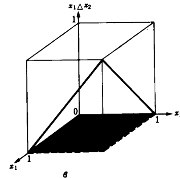
Рис. 2.17. Часто используемые t -нормы.
