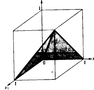
Рис. 2.15. Логическое произведение (x_1 \wedge x_2) .
