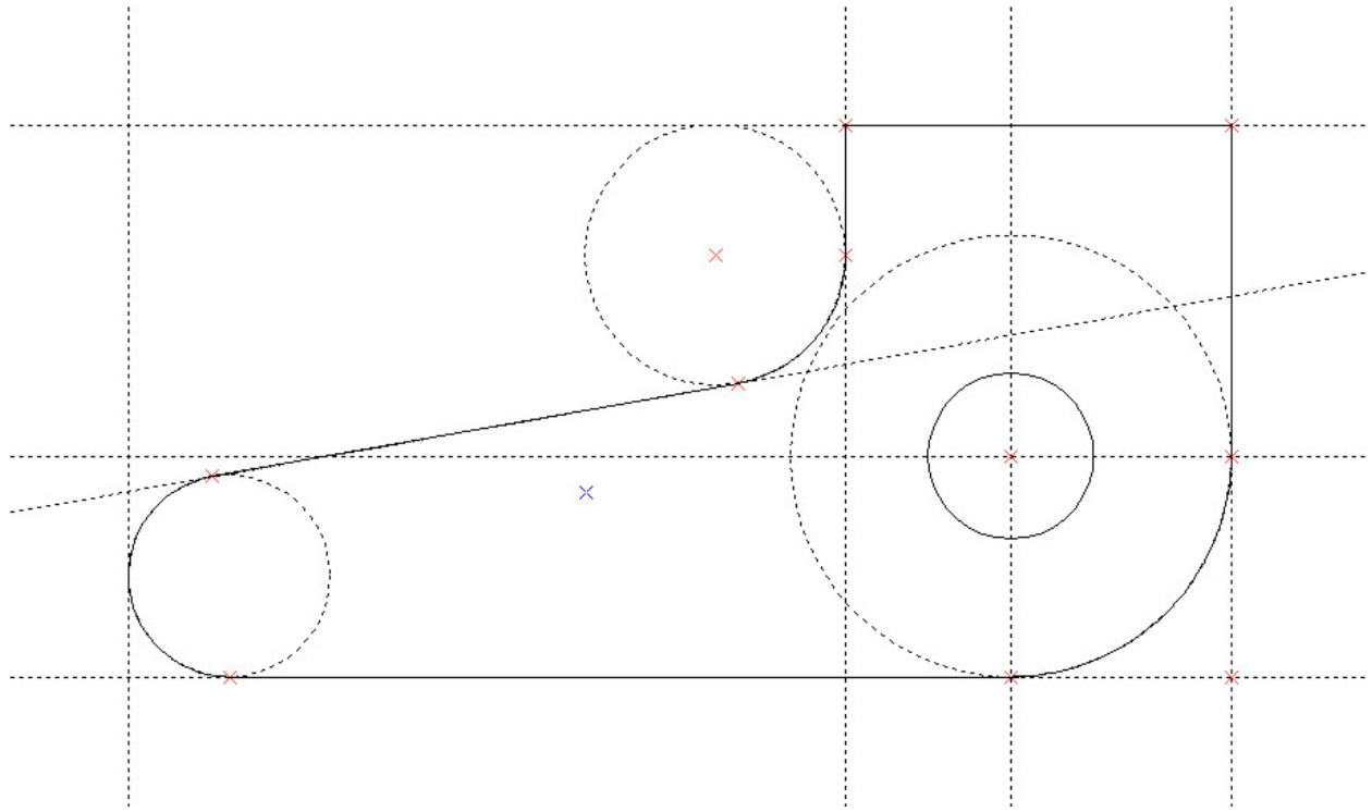
Рис. 21. Построение изображения
