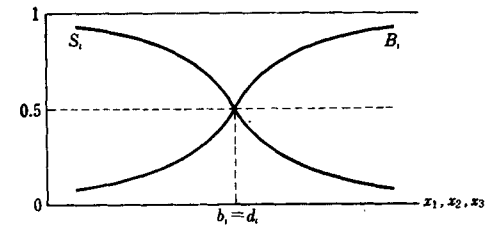
Рис. 3.17. Функция принадлежности.
