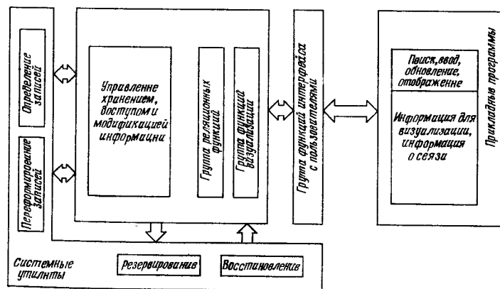
Рис. 4.28. Структура РБД.
