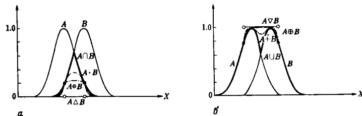
Рис. 2.12. Упорядоченные операции произведения и суммы нечетких множеств.
