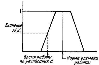
Рис. 4.5. Функция принадлежности.
