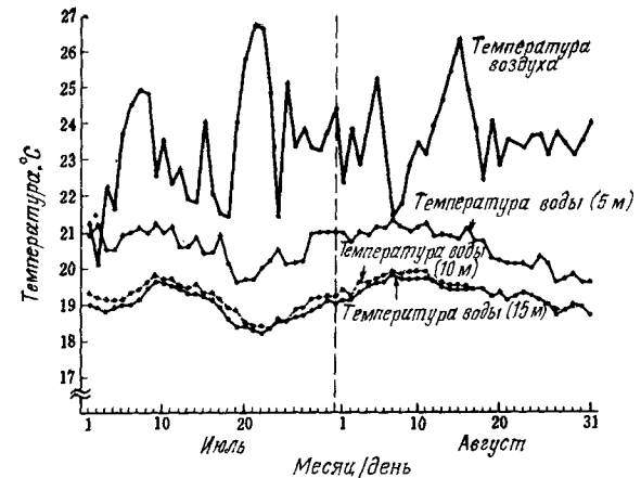
Рис. 5.1. Данные наблюдений.
