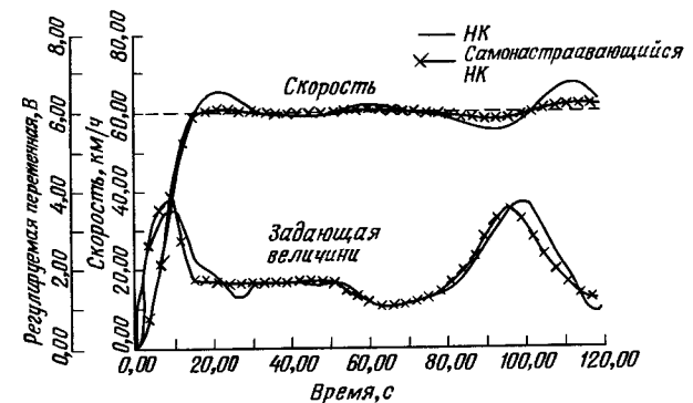
Рис. 3.33. Эффективность управления скоростью с помощью самонастраивающегося НК.
