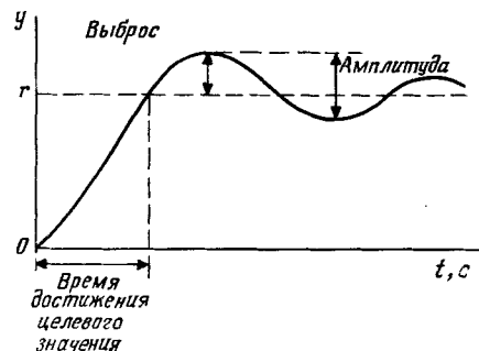
Рис. 3.31. Характеристики управления.
