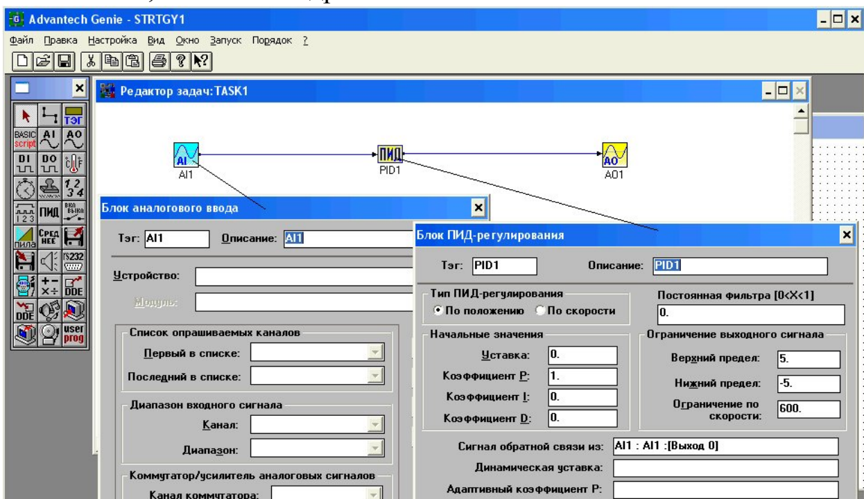
Рис. 34. Задача ПИД-регулятора
