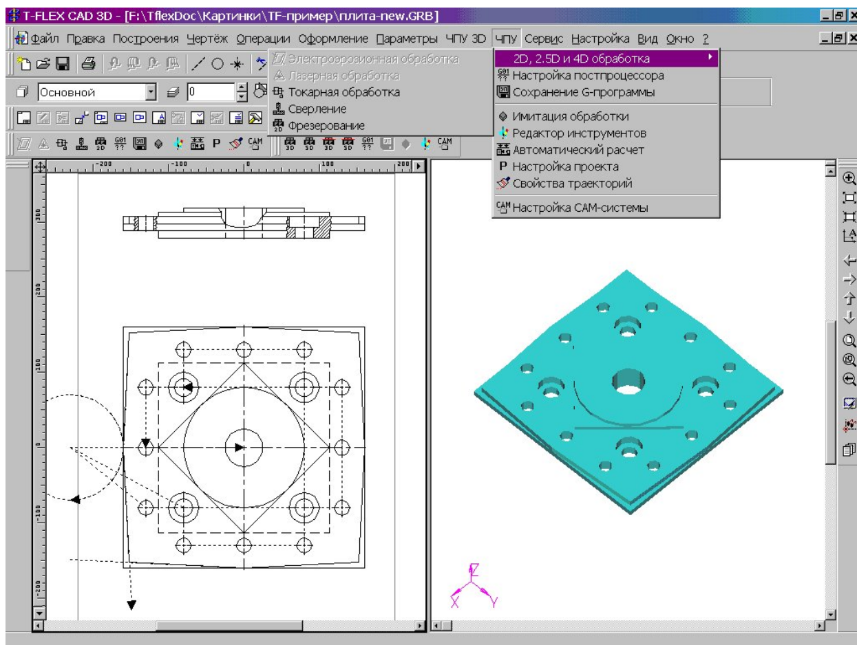
Рис. 25. Вызов T-FLEX/ЧПУ
