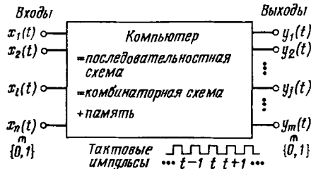
Рис. 2.4. Последовательностная схема.
