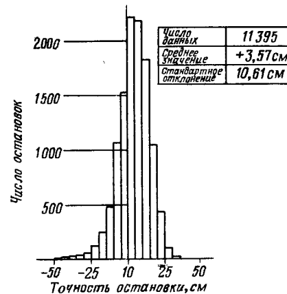
Рис. 3.53. Результаты измерения точности остановки.
