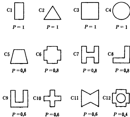
Рис. 3.72. Объекты распознавания.
