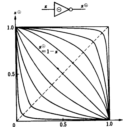
Рис. 2.14. Нечеткие отрицания.
