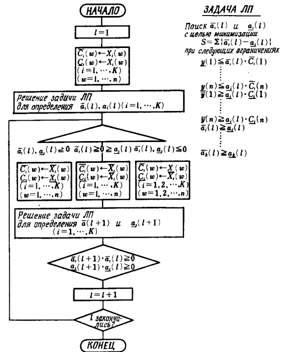
Рис. 5.6. Определение функции нечеткой многоатрибутной оценки.
