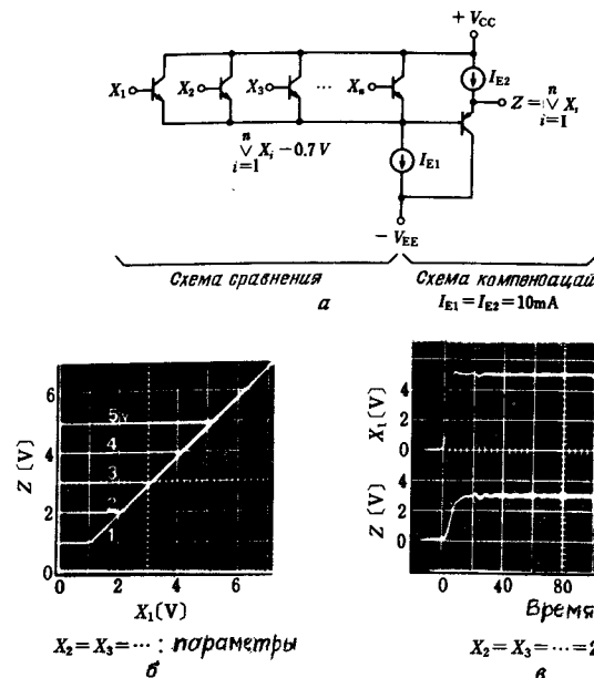
Рис. 6.2. Схема МАХ (а), характеристики входа и выхода (б) и переходная характеристика (в).
