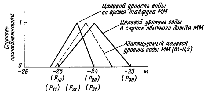
Рис. 3.38. Адаптация функции принадлежности целевого уровня (MM).
