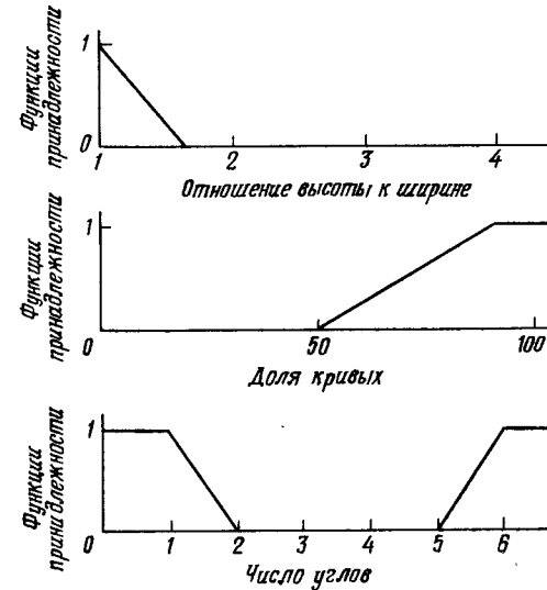
Рис. 3.69. Макропризнаки круга.
