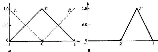
Рис. 2.22. Пример нечеткого вывода по правилам.
