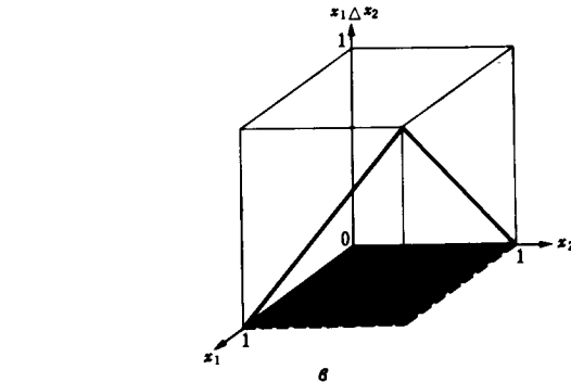
Рис. 2.17. Часто используемые t -нормы.
