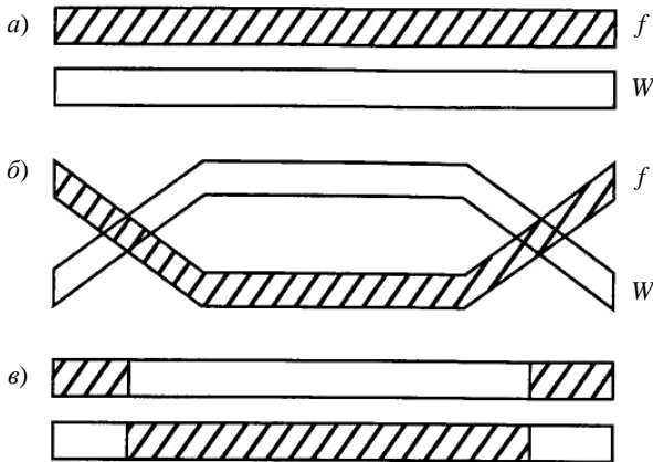
Рис. 3.4. Схема двойного кроссинговера: a – до кроссинговера; б – во время кроссинговера; в – после кроссинговера
