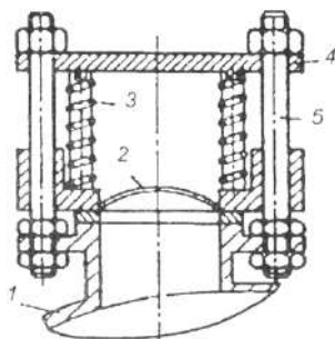
Рисунок 7.2 – Взрывной клапан: 1 – защищаемый сосуд; 2 – запорный диск; 3 – пружина; 4 – кольцо; 5 – штанга
