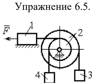
Рис. 6.30. Схема подъёмника
