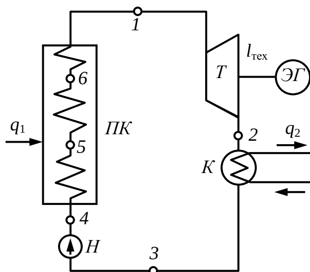
Рис. 3.25. Схема паросиловой установки: ПК – паровой котел; T – паровая турбина; ЭГ – электрогенератор; K – конденсатор; H – насос
