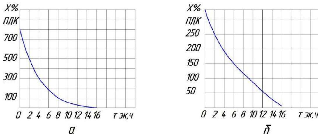
Рисунок 7.1 – Номограммы допустимой экспозиции t_{\text{экз}} от содержания пыли в рабочей зоне: а-нетоксичная пыль, б-токсичная пыль
