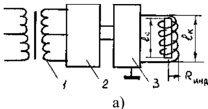
Рис 4.1 Схема генератора для нагрева металла (а) и неметаллич. материалов (б)
