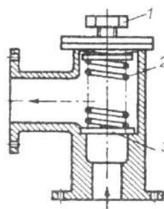
Рисунок 7.3 – Пружинный клапан: 1 – регулировочный винт; 2 – пружина; 3 – клапан
