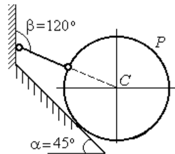
Рис. 1.7. Равновесие шара
