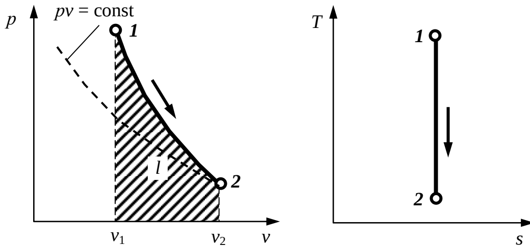
Рис. 3.14. Адиабатный процесс
