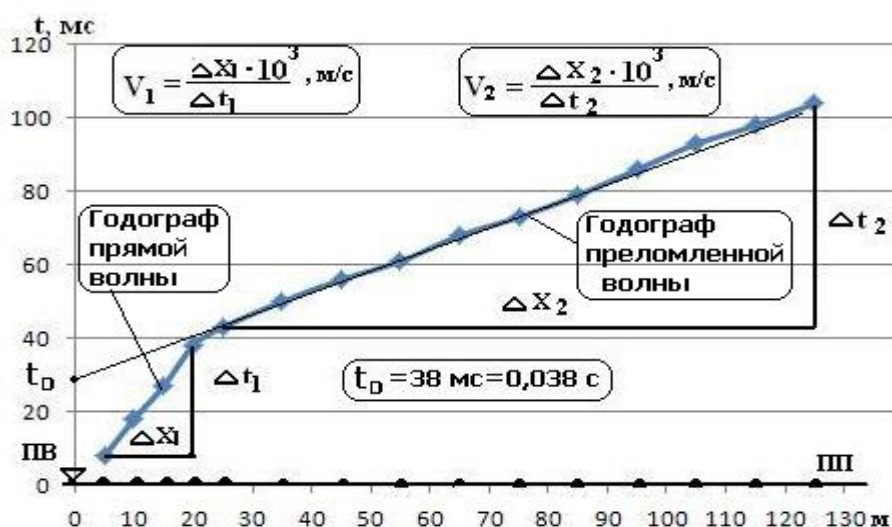
Рис. 3.3. Годографы прямой и преломленной волн. V_1=500 \text{ м/с} , V_2=1670 \text{ м/с} , критический угол i=\arcsin(V_1/V_2)=17,5^\circ . Мощность первого слоя h_1=20 \text{ м} (формула расчёта приведена в тексте)
