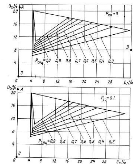
Рис. 1. Треугольники взрываемости
