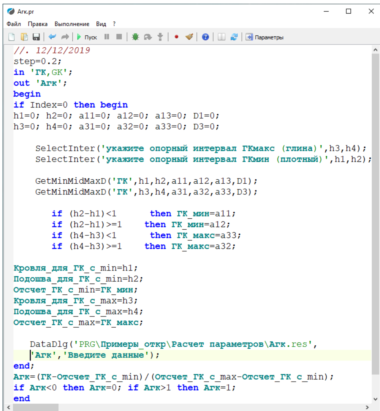
Рис. 2.30. Программа расчета параметра Агк
