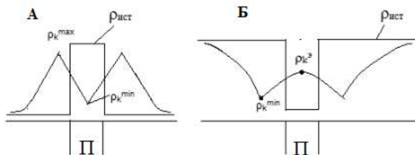
Рис. 5.5. Пример графиков \rho_k (потенциал – зонд АМ) и истинного УС ( \rho^{\text{ист}} ) для среды с тонким прослоем (П) относительно повышенного и пониженного УС при его мощности h=0,5\text{AM}
