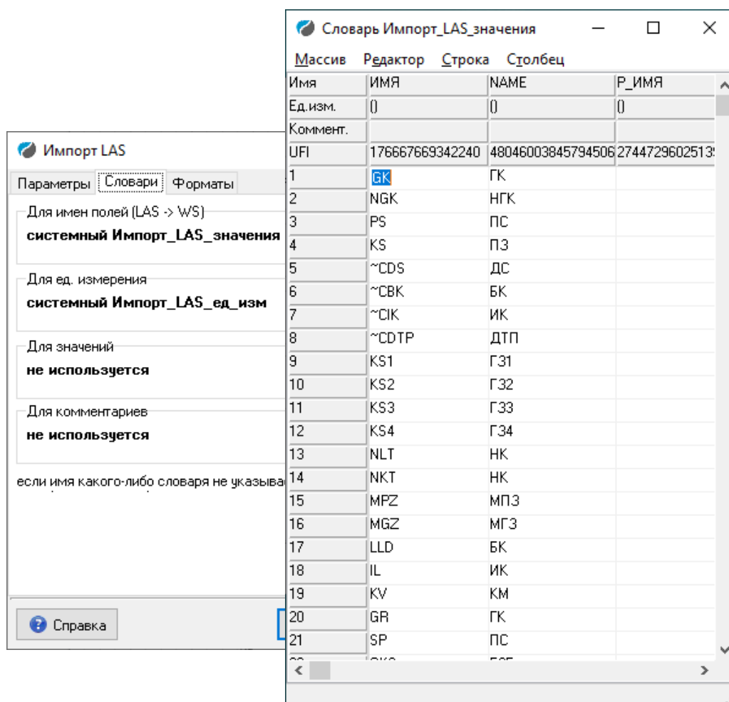
Рис. 2.10. Редактирование системного словаря
