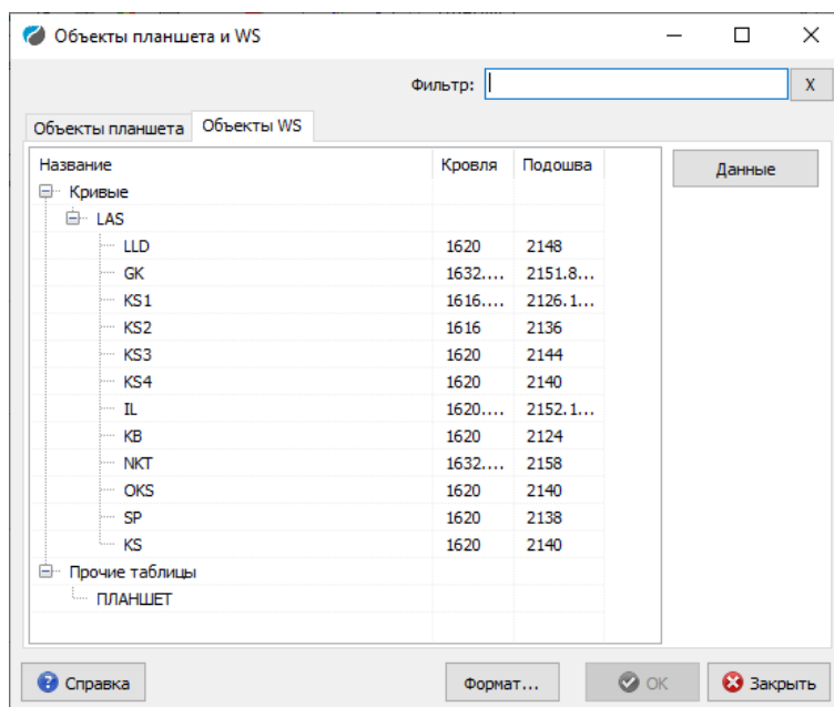
Рис. 2.912 Список объектов планшета
