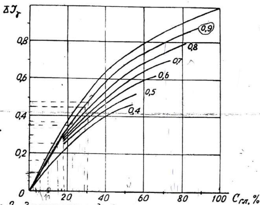
Рис. 2. Зависимость двойного разностного параметра от глинистости. Шифр кривых - C_{гг} опорного горизонта
