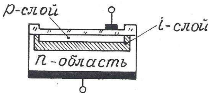
Рис. 3.9. Структура pin-диода
