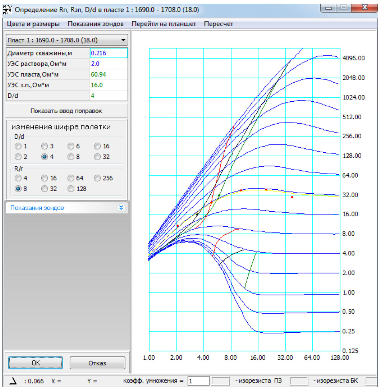
Рис. 2.44. Палетка для определения УЭС
