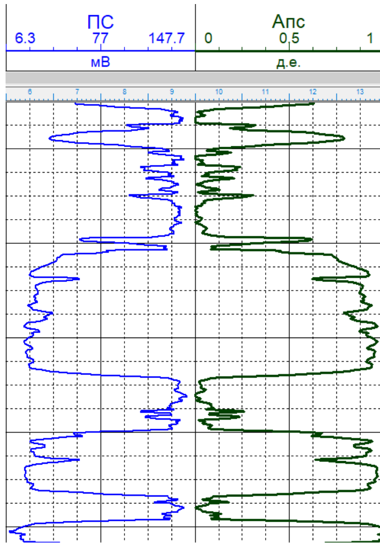
Рис. 2.27. Формы кривых ПС и Апс
