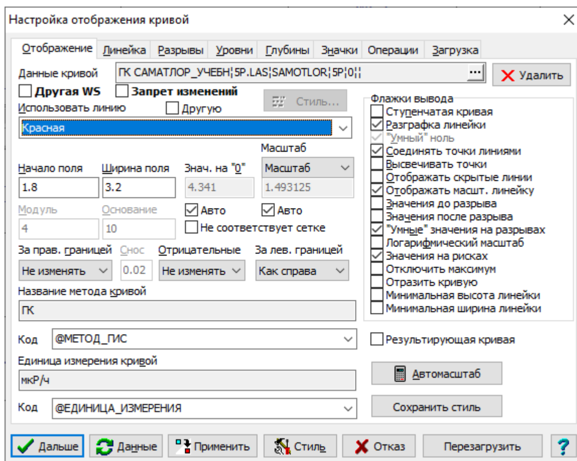
Рис. 2.17 Окно свойств кривой
