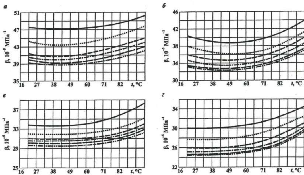
Рис. 87. Зависимость сжимаемости водных растворов NaCl от минерализации, температуры и давления (В.М. Добрынин, 2000): a-г – C_s соответственно 0, 100, 200 и 300 г/л
