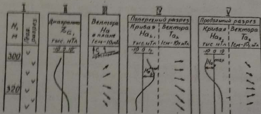
Рис. 41. Пример изображения результатов скважинной трех-компонентной магнитотеллурки
