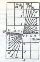
Рис. 29. Номограмма для определения индукционного параметра P (шифр приклад-1).
