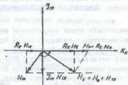
Рис.19 Векторная диаграмма магнитного H_0 , индуцированного H_a и результирующего H_c магнитных полей.
