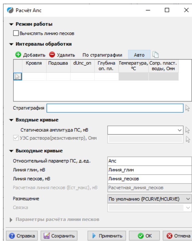
Рис. 2.24. Автоматическое определение интервала обработки
