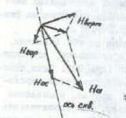
Рис.20 Векторная диаграмма пространственных компонент магнитного поля.
