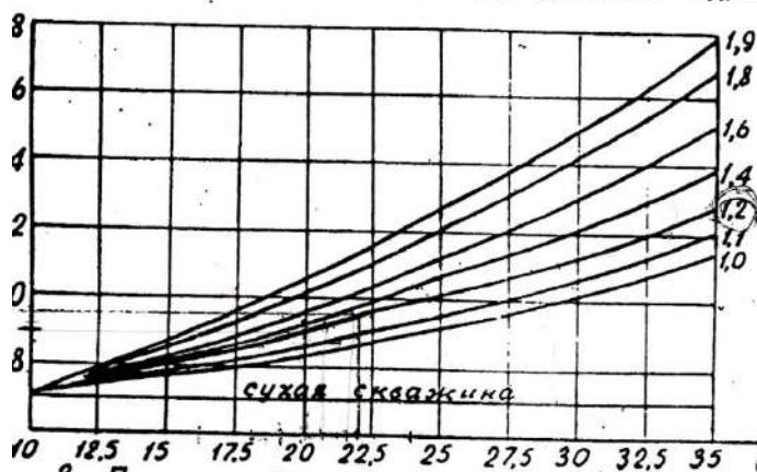
Рис. 2. Зависимость двойного разностного параметра от глинистости. Шифр кривых - C_{гг} опорного горизонта
