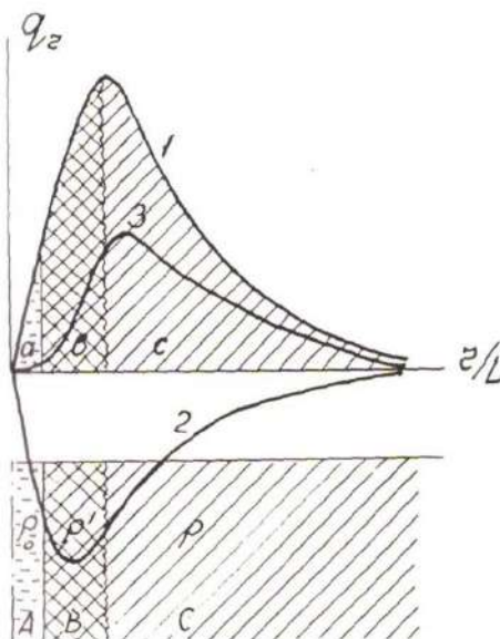
Рис. 2. Радиальный геометрический фактор 1-двухкатушечного зонда КГ-КГ, 2-додолькифельного зонда ФГ-КП, 3-трехкатушечного зонда
