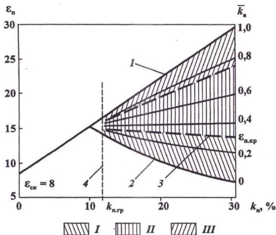
Рис. 44. Зависимость \varepsilon_n = f(k_n) :
