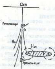
Рис.18 Распределение силовых линий первичного ( H_0 ) и индуцированного ( H_a ) магнитного поля.
