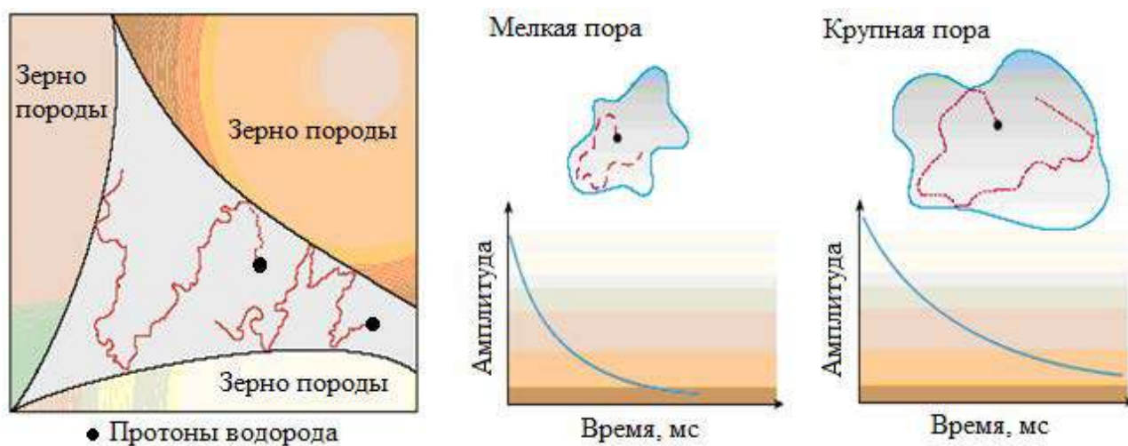
Рис. 7.6. Поверхностная релаксация.
