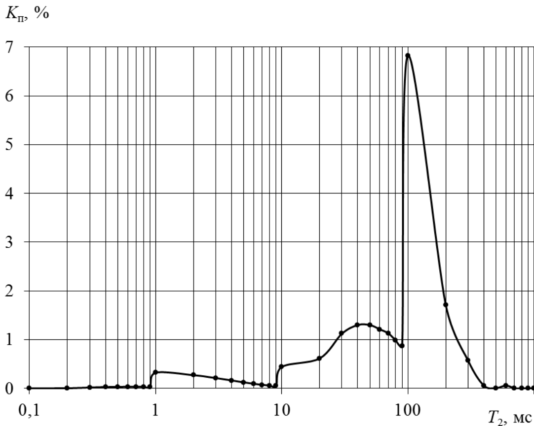
Рис. 7.13. Парциальный спектр
