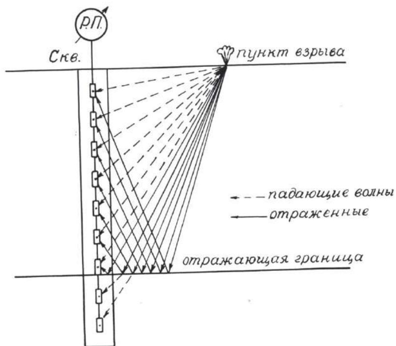
Рис. 1. Типовая схема наблюдений в ВСП.
