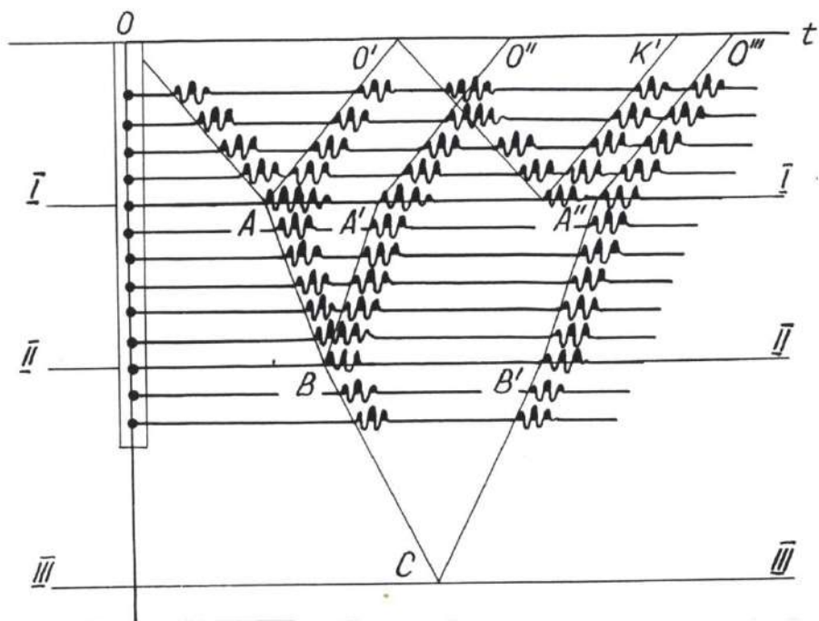
Рис. 2. Сейсмограммы прямых и отраженных волн при типовой схеме наблюдений ВСП.
