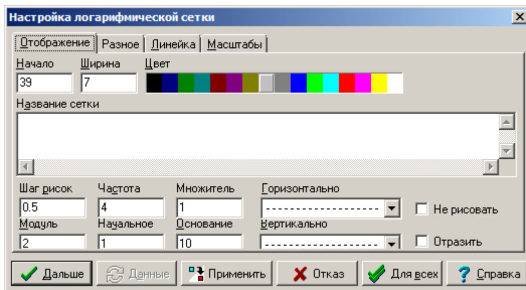
Рис. 1.8. Настройка параметров сетки
