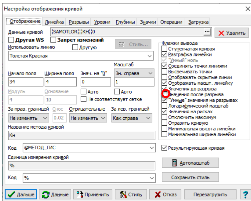
Рис. 2.50. Свойства кривой Кн
