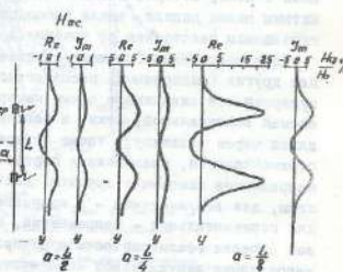
Рис.22 График осевой компоненты аномалии от расстояния пластины при разных расстояниях ( a ) пластины от скважины.
