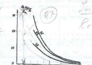
Рис.23 Зависимость пространственной аномалии от расстояния пластины от скважины и угла падения. Штриховая линия - I_m H_a / I_0 H_0 .
