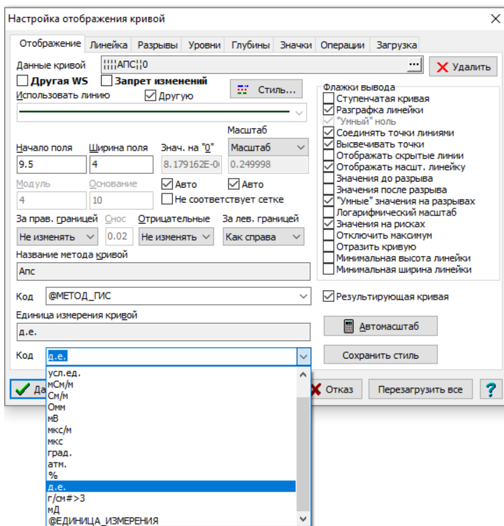
Рис.2.26. Настройка единиц измерения кривой Апс
