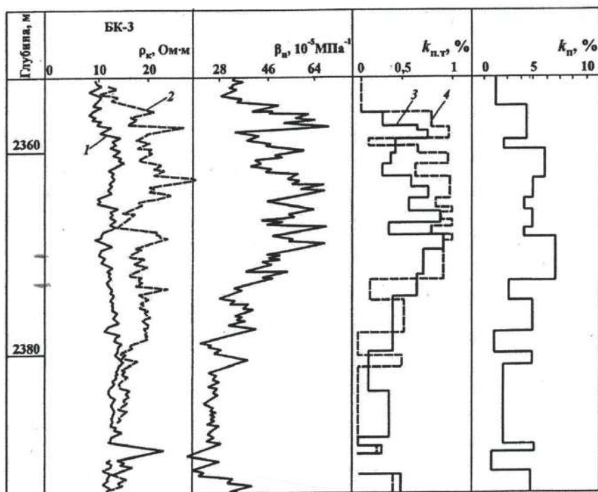
Рис. 89. Определение k_{п.т} по данным АКШ в порово-трещинном коллекторе (карбонатный разрез). Кривые \rho_k : 1 – \rho_p = 0,5 \text{ Ом}\cdot\text{м} , 2 – \rho_p = 2,4 \text{ Ом}\cdot\text{м} ; графики k_{п.т} , построенные по данным методов: 3 – двух растворов, 4 – АКШ (по В.А. Костериной)
