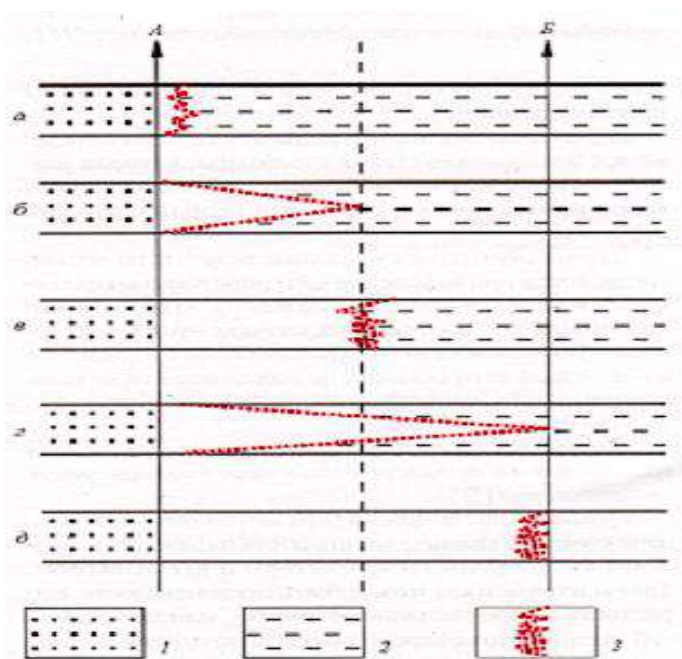
Рис. 3.3. Модели замещения коллекторов в межскважинном пространстве скважин А (скрывшей коллектор) и В (пробуренной в зоне отсутствия коллектора)
