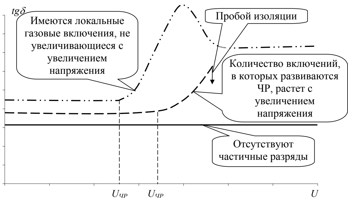
Рис. 6.19. Характерные зависимости \text{tg}\delta от величины испытательного напряжения, где U_{\text{чр}} - напряжение возникновения частичных разрядов.
