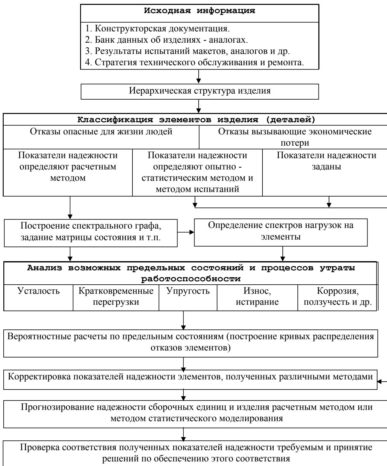
Рис. 3.1. Блок - схема прогнозирования надежности изделий при проектировании
