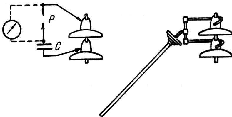
Рис. 6.25. Схема испытания многоэлементных изоляторов при помощи специальной штанги.
