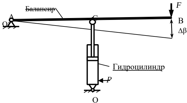
Рис. 1. Расчетная схема
