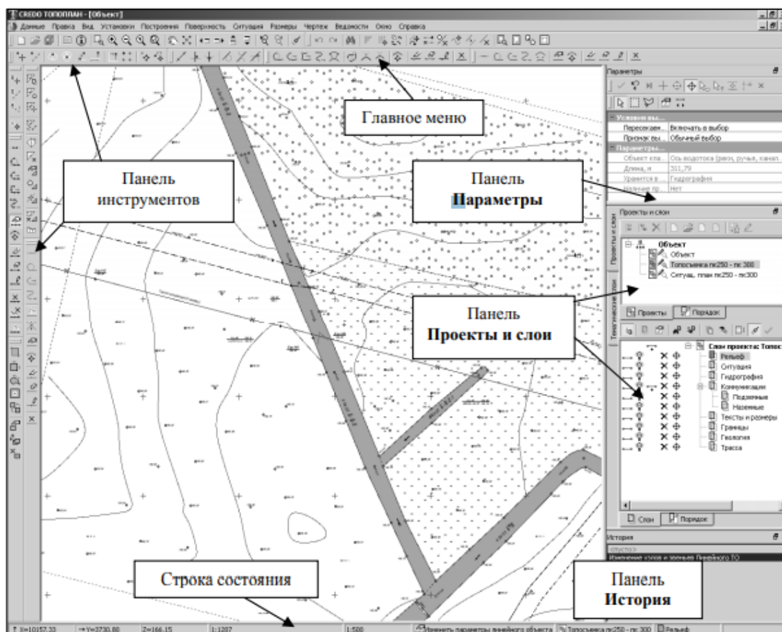
Рис. 3.1. Интерфейс программы «Объем»
