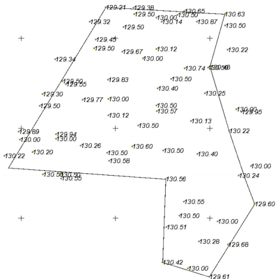
Рис. 3.15. Рельефные точки проекта
