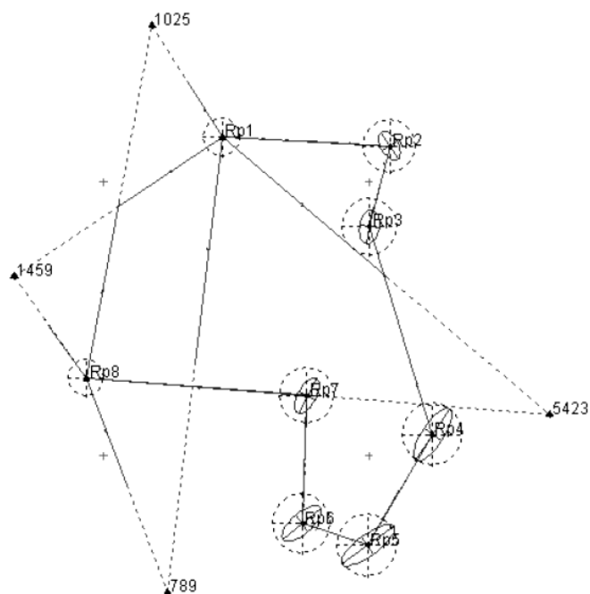
Рис. 1.9. Совместное уравнивание сети
